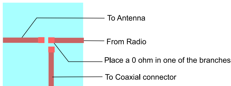
Figure 56. 支线示例
