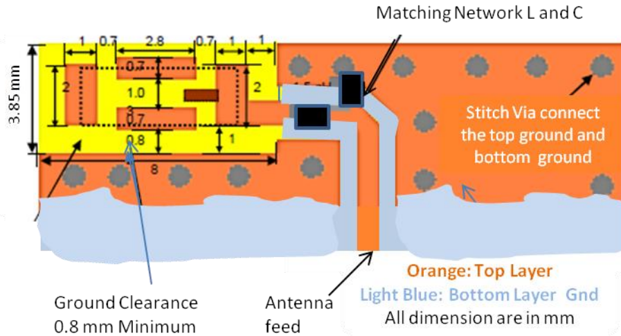
Figure 20. 具有约翰森技术的 2450AT42B100E 芯片天线的布局指南
