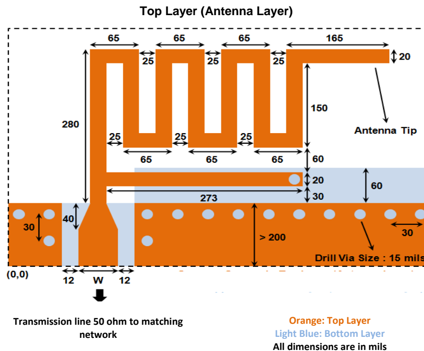
Figure 10. MIFA 布局
