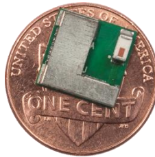
Figure 6. 带芯片天线的 Cypress EZ BLE 模块 (10 mm x 10 mm)
