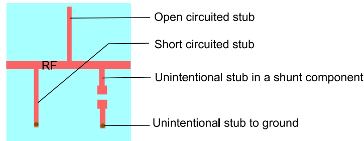
Figure 29. 短截线示例
