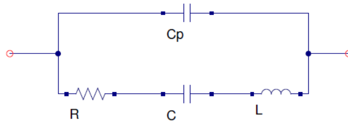
Figure 54. 电容器模型
