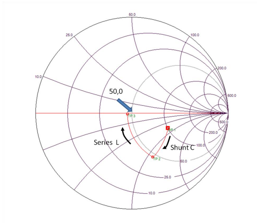
Figure 42. 在 Smith 图表中转换为 50 Ω
