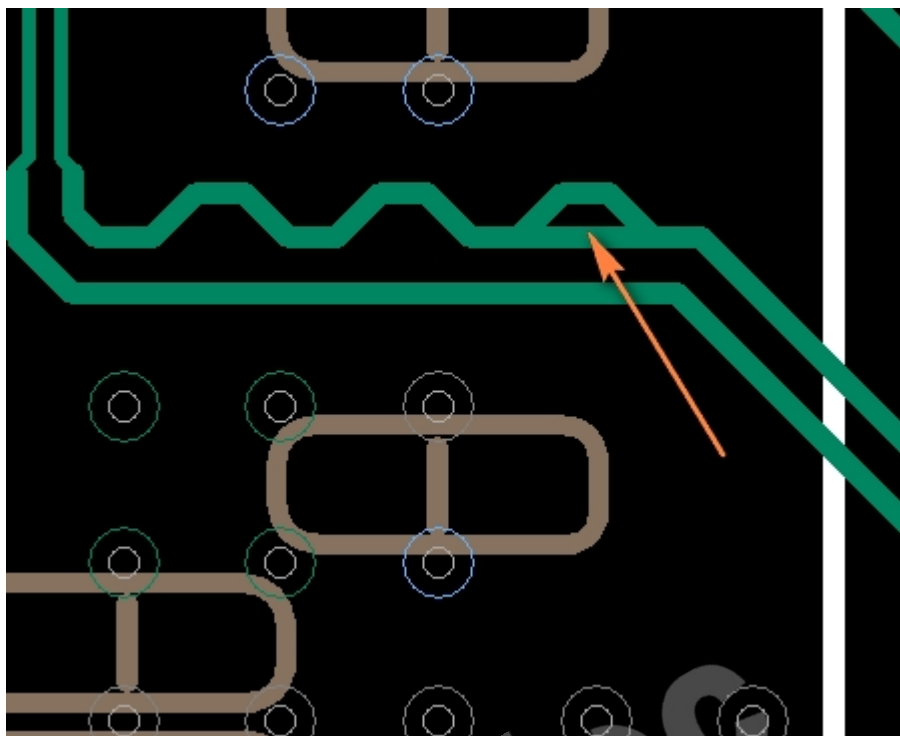
走线到焊盘间距过近，差点接吻了。
