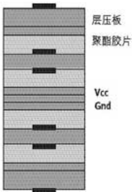
图 2: 优秀设计方案的第一步是正确设计叠层结构
